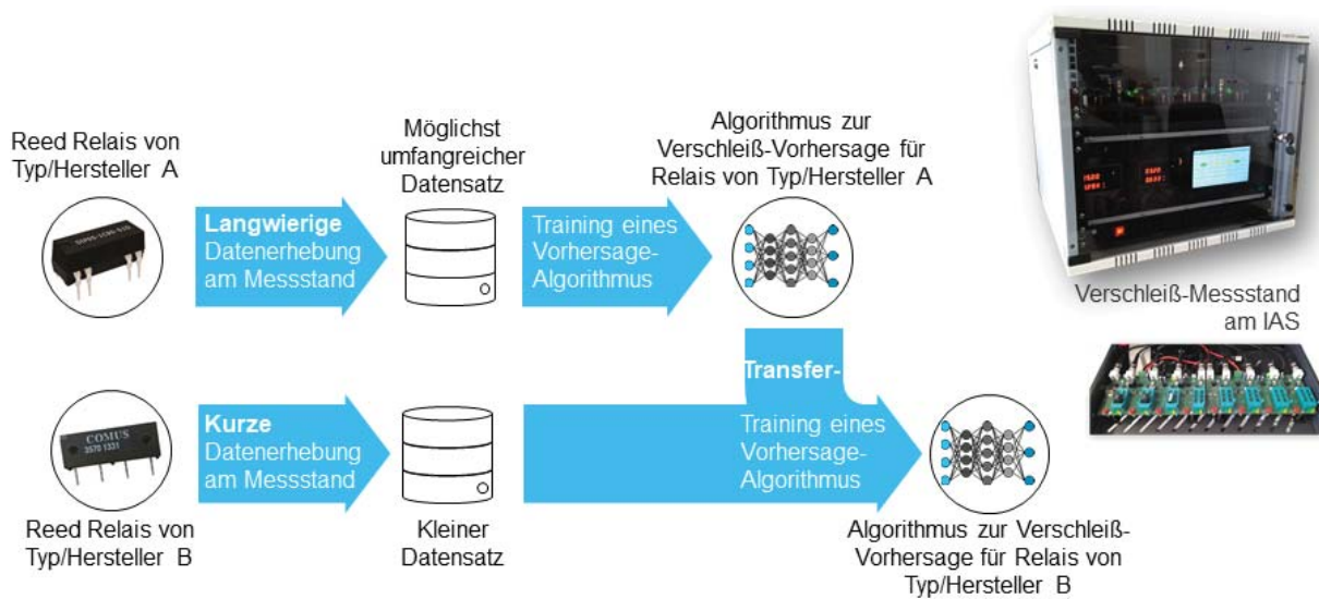
Beispiel-Anwendung für industrielles Transfer-Lernen: Verschleißvorhersage für Reed-Relais über verschiedene Typen/Hersteller hinweg
